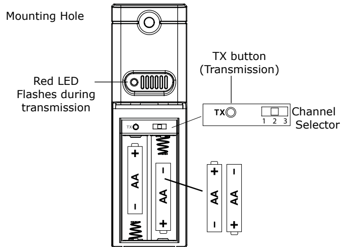
Optional Add-on TX141TH-BCH Sensor
